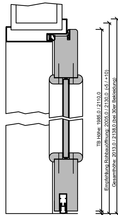
114-400-100-304-Höhenschnitt.dwg
