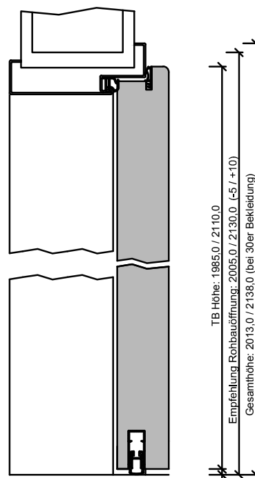
105-400-100-304-Höhenschnitt.dwg
