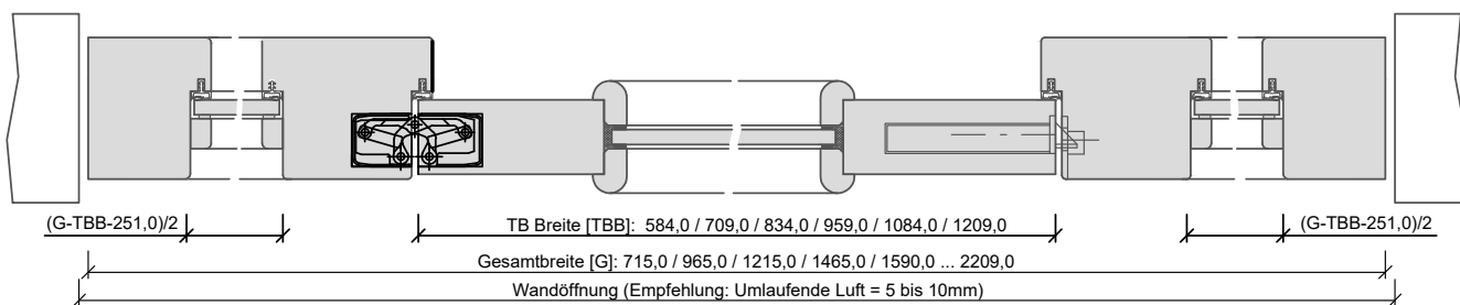
Q_RD_TB-BLO-1FLG_WF2_STU_RD-40-LA.dwg
