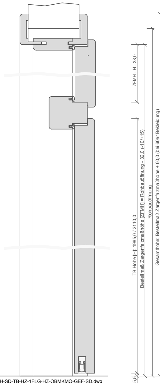
G-H-SD-TB-HZ-1FLG-HZ-OBKMQ-GEF-SD.dwg
