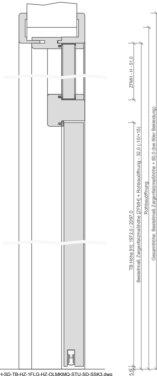
G-H-SD-TB-HZ-1FLG-HZ-OLMKMQ-STU-SD-SSK3.dwg
