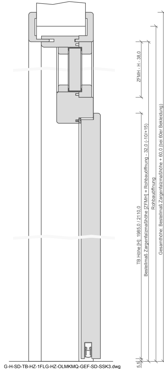
G-H-SD-TB-HZ-1FLG-HZ-OLMKMQ-GEF-SD-SSK3.dwg
