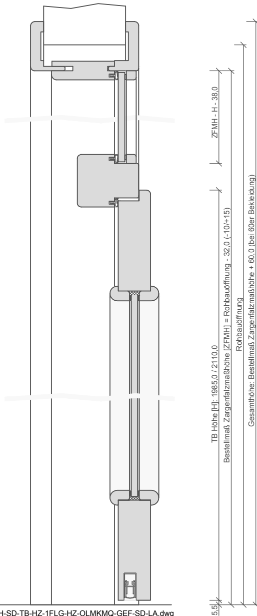
G-H-SD-TB-HZ-1FLG-HZ-OLMKMQ-GEF-SD-LA.dwg
