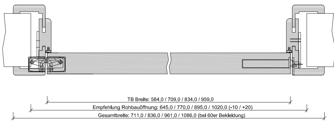
200-800-103-100-Querschnitt.dwg
