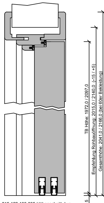
215-122-100-305-Höhenschnitt.dwg
