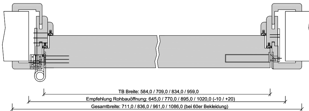
226-226-108-100-Querschnitt.dwg
