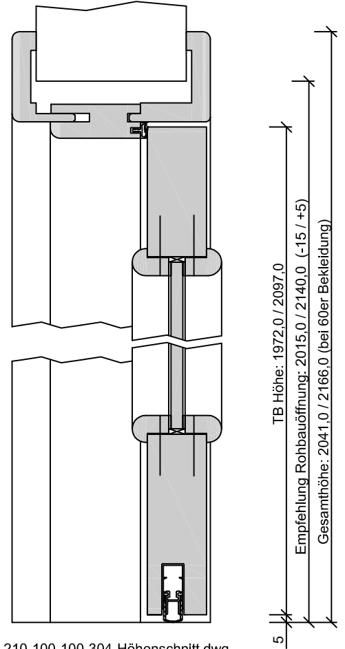
210-100-100-304-Höhenschnitt.dwg
