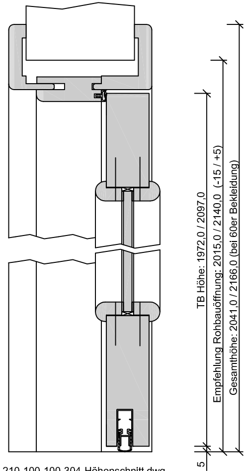
210-100-100-304-Höhenschnitt.dwg
