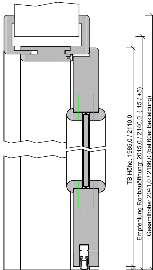
110-100-100-304-Höhenschnitt.dwg
