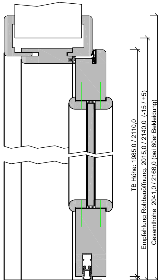
114-100-100-304-Höhenschnitt.dwg
